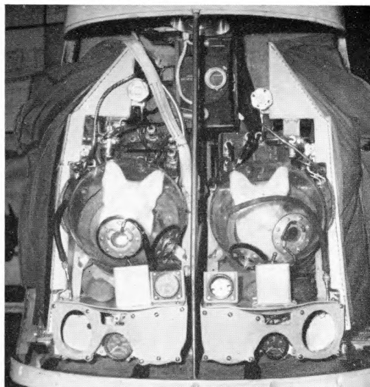
The Strelka/Belka capsule
