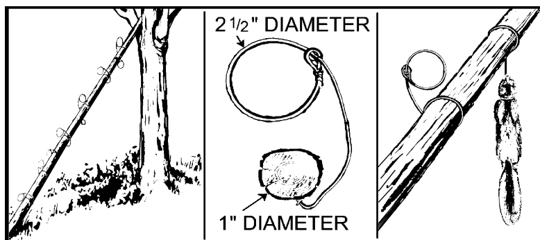
Figure VIII-4. Squirrel Pole
