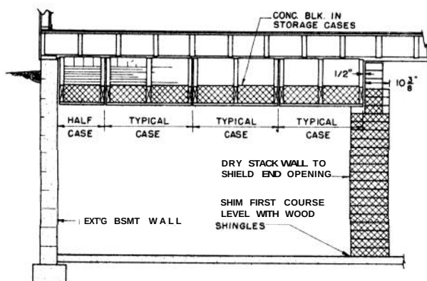
SECTION A-I
